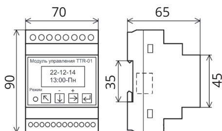
Внешний вид и габаритные размеры TTR-01
