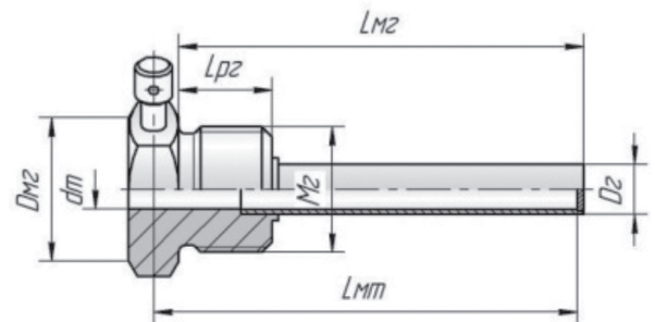
ГЦР.105 для ТП с клеммной головкой
