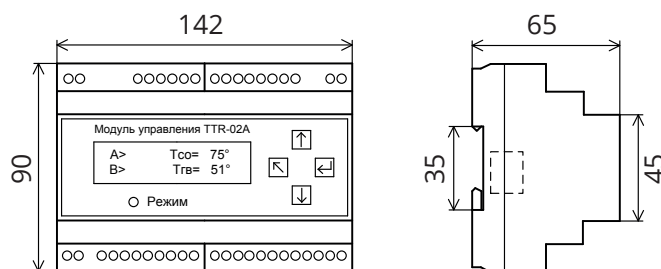
Внешний вид и габаритные размеры TTR-02
